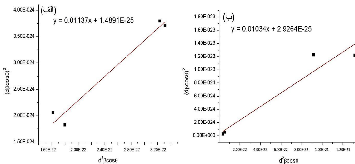
شکل ۲: نمودارهای رگرسیون سایز – استرین مدل نانوکریستال‌های WO_3 کلسینه شده در دماهای (الف) ۴۰۰ و (ب) ۴۵۰ درجه سانتی‌گراد
