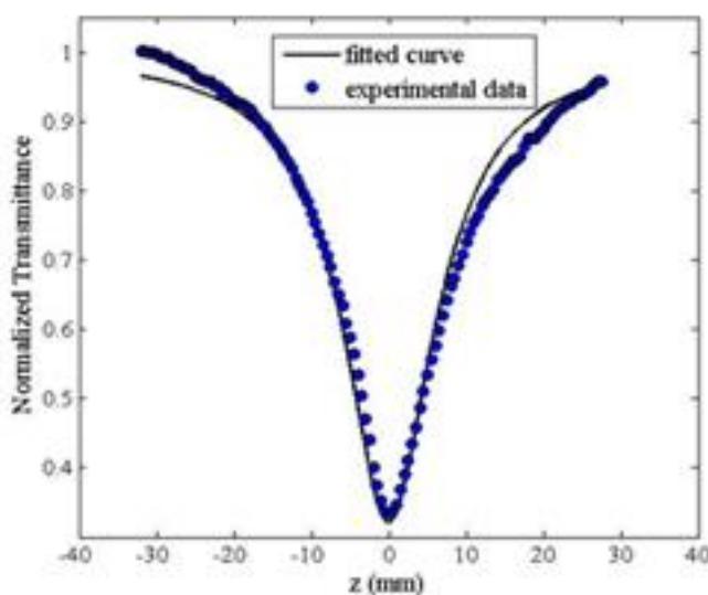
شکل ۴. حالت روزنه باز روبش خطی نانوذرات نقره با غلظت 3 \times 10^{-3} \times 2/94
