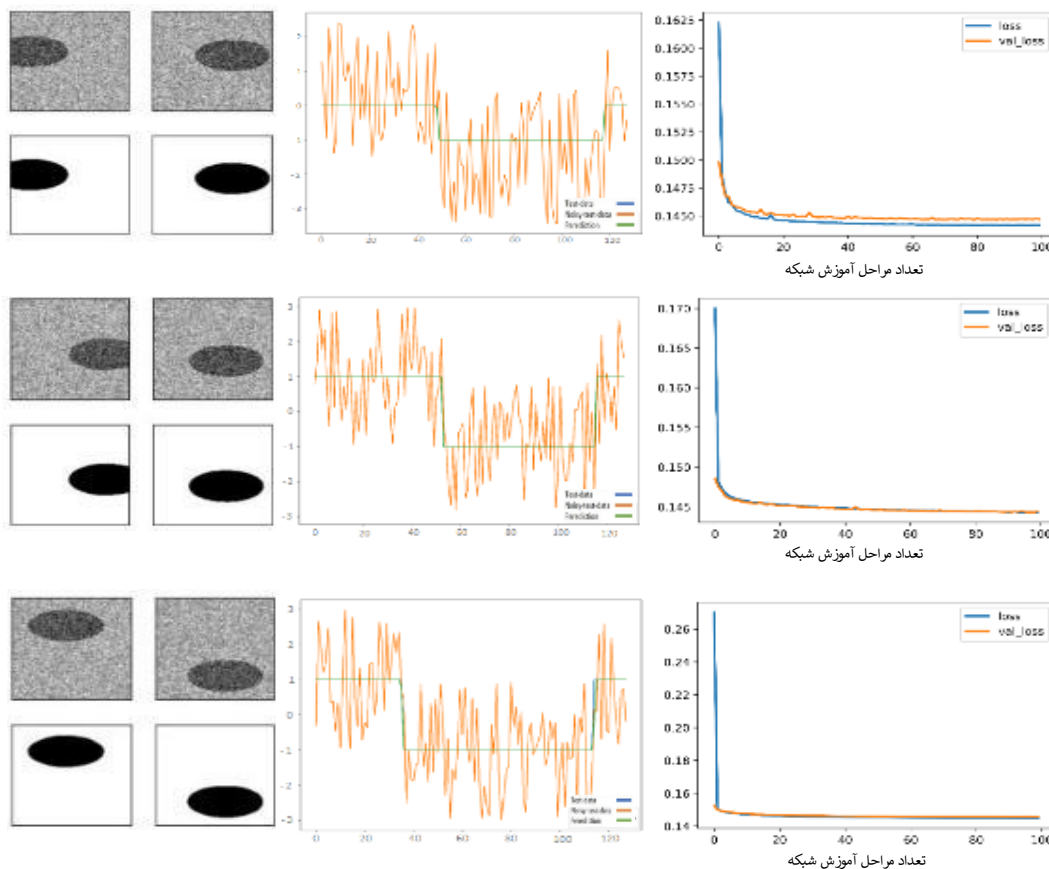
شکل ۷ نمونه‌ای از داده‌های نوع دوم همراه با نویز و نسخه‌ی رفع نویز شده، همراه با مقایسه‌ی برش عرضی داده‌ها و خطای حاصل از فرآیند حذف نویز. نتایج از بالا به پایین به ترتیب مربوط به نرخ‌های یادگیری ۰/۰۱، ۰/۰۰۱ و ۰/۰۰۰۱ هستند.
