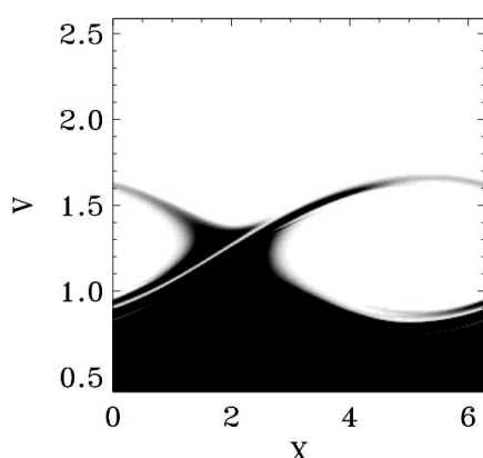
شکل ۴. تصویری از فضای فاز کلاسیک تابع توزیع الکترون در ناحیه اطراف سرعت فاز موج. موقعیت بر حسب \lambda_F و سرعت بر حسب v_F نرمال‌سازی شده‌اند. پارامترهای شبیه‌سازی عبارتند از: T = 0.01T_F و \alpha = 0.1 و k\lambda_F = 1
