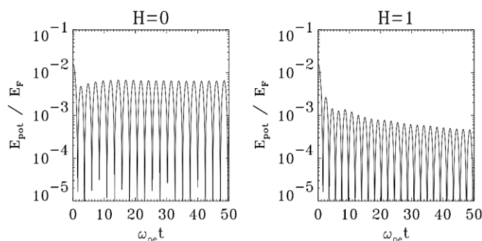
شکل ۶. تغییرات زمانی انرژی پتانسیل، که نسبت به انرژی فرمی نرمال‌سازی شده است، برای حالت کلاسیک (در چارچوب چپ) و حالت کوانتومی با H = 1 (در چارچوب راست) نمایش داده شده است.
