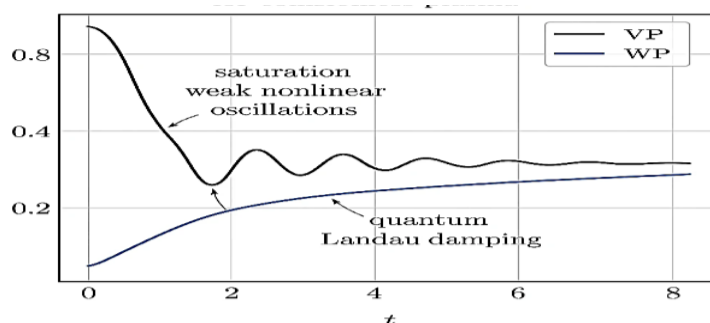
شکل ۷. تکامل زمانی دامنه میدان الکتریکی |E_k(t)| در پلاسمای بی‌برخورد برای مدل‌های ولاسوف-پواسون (VP) و ویگنر-پواسون (WP). در مدل VP، میرایی اولیه به اشباع غیرخطی منجر شده در حالی که در مدل WP، میرایی به‌صورت یکنواخت‌تر ادامه یافته است.
