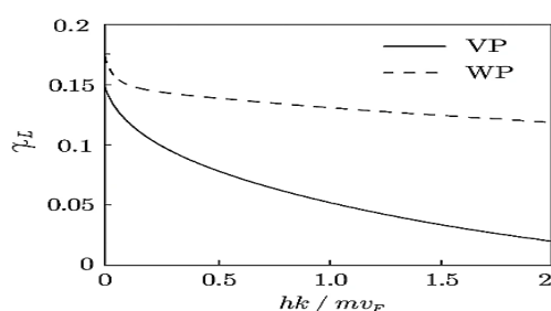
شکل ۸. نرخ میرایی لاندائو \gamma_L بر حسب پارامتر کوانتومی \frac{\hbar k}{m v_F} برای مدل‌های ولاسوف-پواسون (VP) و ویگنر-پواسون (WP)
