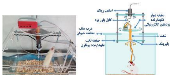
شکل ۱۲: طراحی و ساخت سیستم روتاری کانکتور برای جلوگیری از پیچش کابل‌های ایمپلنت بر روی محفظه حیوان.
