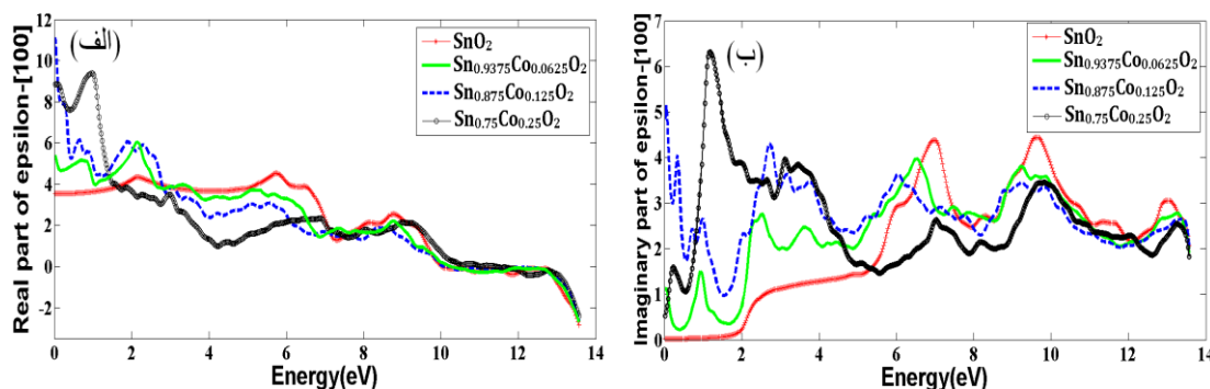
شکل ۱۲: نمودار تابع دی‌الکتریک بر حسب انرژی برای نمونه \text{Sn}_{1-x}\text{Co}_x\text{O}_2 در راستای [100] ، (الف) بخش حقیقی
