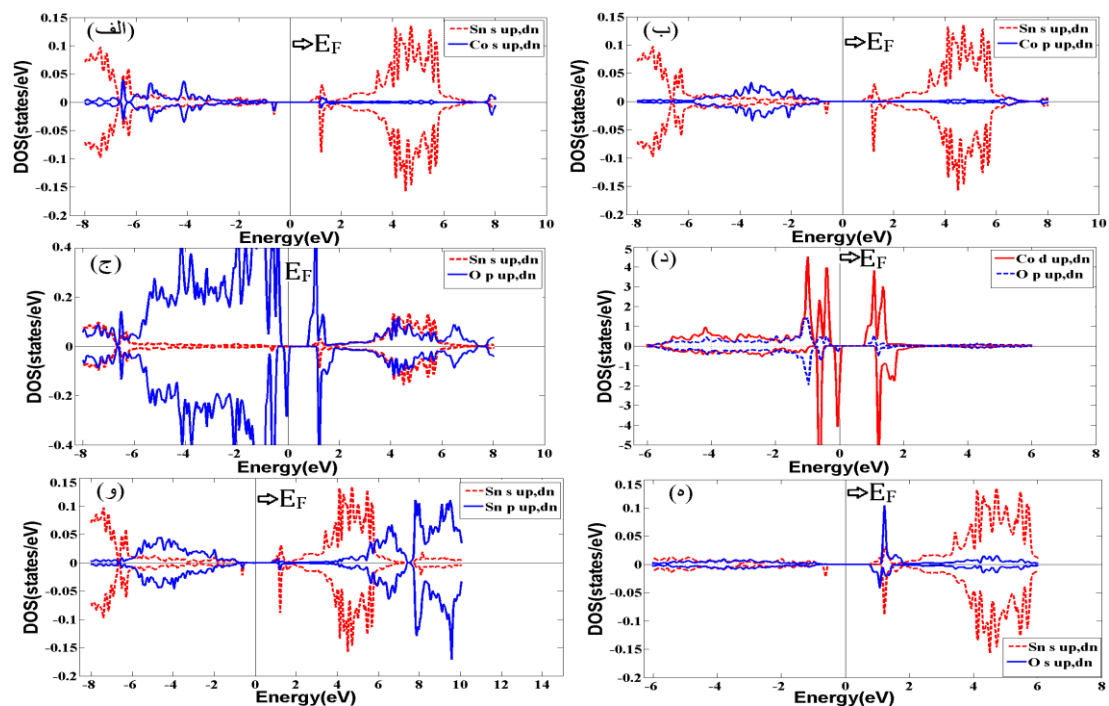
شکل ۳: نمودار مربوط به چگالی حالت‌های جزئی عناصر نمونه \text{Sn}_{0.9375}\text{Co}_{0.0625}\text{O}_2 . الف) \text{Sn s up,dn} ، \text{Co s up,dn} ، ب) \text{Sn s up,dn} ، \text{Co p up,dn} ، ج) \text{Co p up,dn} ، \text{O p up,dn} ، د) \text{Co d up,dn} ، \text{O p up,dn} ، ه) \text{Sn p up,dn} ، \text{Sn s up,dn} و \text{O s up,dn} .
