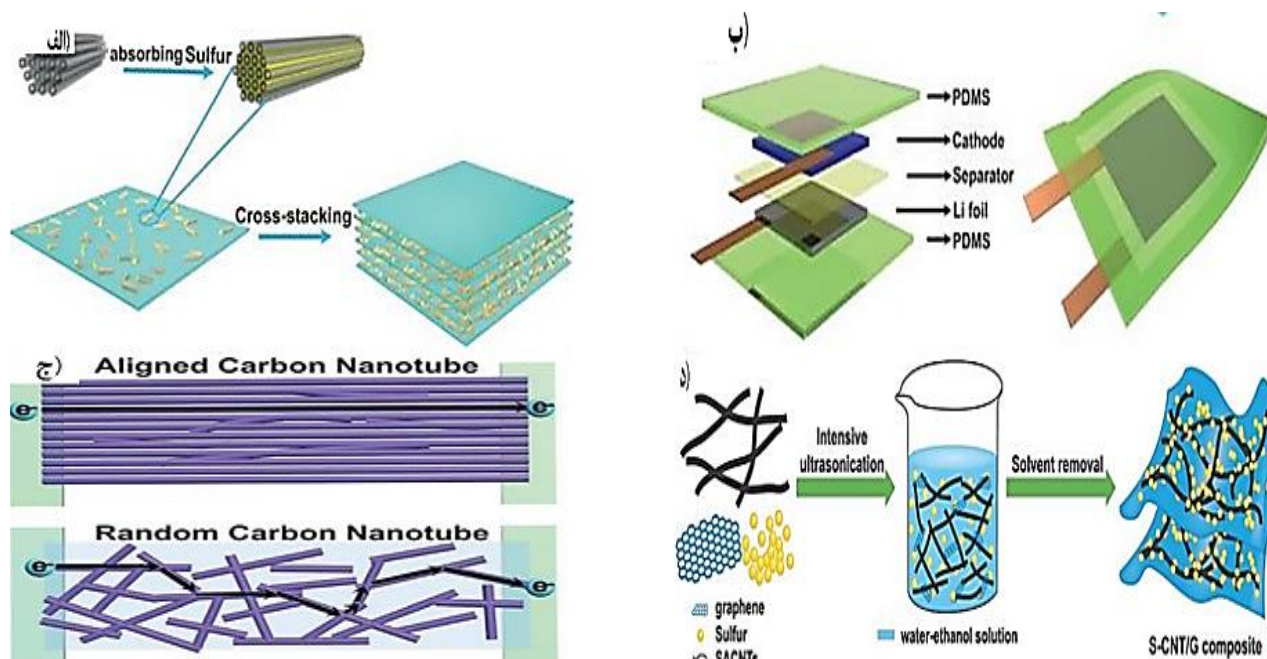
شکل ۱. (الف) فرآیند ساخت کاتد سولفور هیبریدی چندلایه و (ب) تصویر شماتیک از ساختار باتری Li-S انعطاف پذیر. (ج) مقایسه برای توضیح تفاوت‌های رسانایی الکترونیکی بین CNTهای تراشده و CNTهای تصادفی [۲۳]. حق چاپ ۲۰۱۵، John Wiley & Sons. (د) روش آماده سازی برای سنتز S-CNT/G [۲۴]. حق چاپ ۲۰۱۵، Royal Society of Chemistry.
