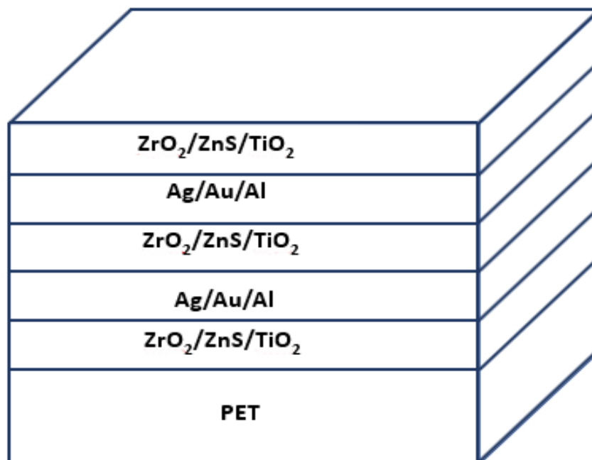
شکل ۱: شماتیک اولیه ساختار الکتروکود رسانای شفاف
