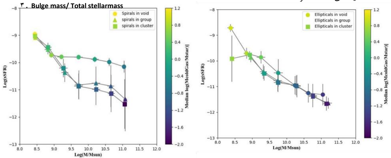
شکل ۳. مقایسه sSFR - جرم ستاره ای کهکشانها در محیطهای مختلف. این نرخ بالای تشکیل ستاره در کهکشانهای واقع در تپه جا را می توان به مقدار بیشتر گاز سرد (ستاره ساز) موجود در این کهکشانها نسبت داد.
