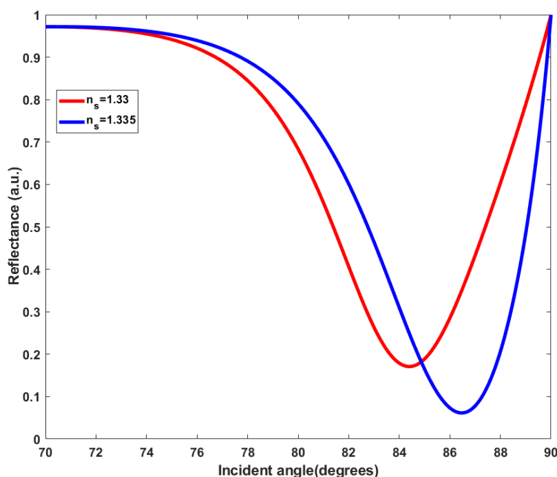
شکل ۶: بازتاب نور ساختار CaF_2 / Ag\ 31\ nm / Ni\ 4\ nm / WS_2\ 1L
