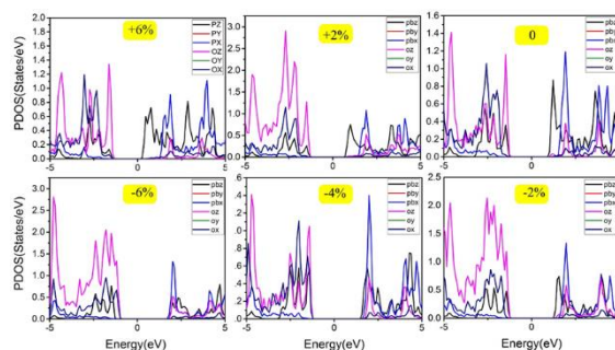
شکل ۱۰- نمودار تغییرات چگالی حالات جزئی برای کرنش دو محوره
