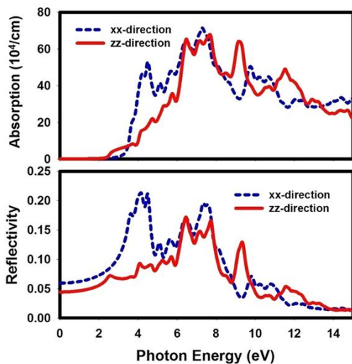
شکل ۹- قسمت حقیقی و موهومی تابع دی‌الکتریک مختلط برای تک لایه \alpha -PbO (بالا) و بازتاب (پائین) برای فوتون‌های ورودی عمود بر سطح (ZZ جهت)، و موازی سطح (XX جهت)
