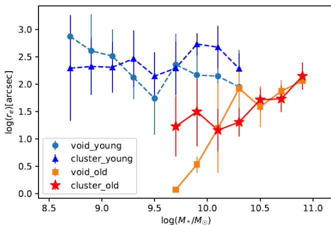
شکل ۳. نمودار تغییرات اندازه کهکشان (شعاع مؤثر) برحسب جرم ستاره‌ای کهکشان‌های پیر و جوان در دو محیط مختلف
