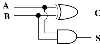
شکل (۱) مدار نیم جمع کننده
