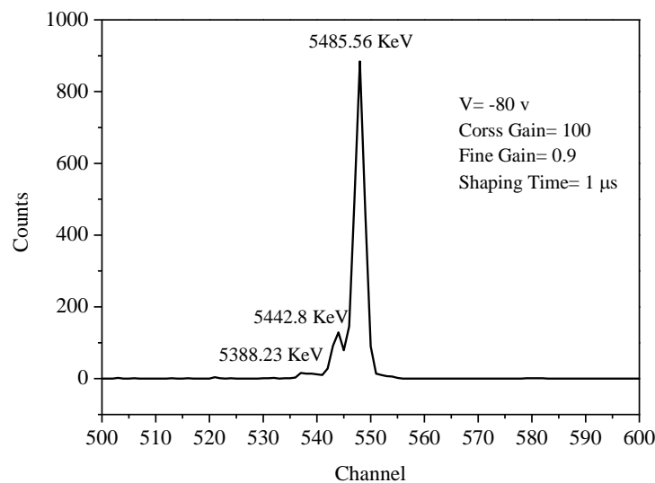
شکل ۷. طیف ذرات آلفای ۵/۴۸ MeV از چشمه‌ی ^{241}\text{Am} آشکارشده توسط آشکارساز سیلیکونی PIN دایروی با مساحت 163 \text{ mm}^2 تحت ولتاژ معکوس ۸۰ V.
