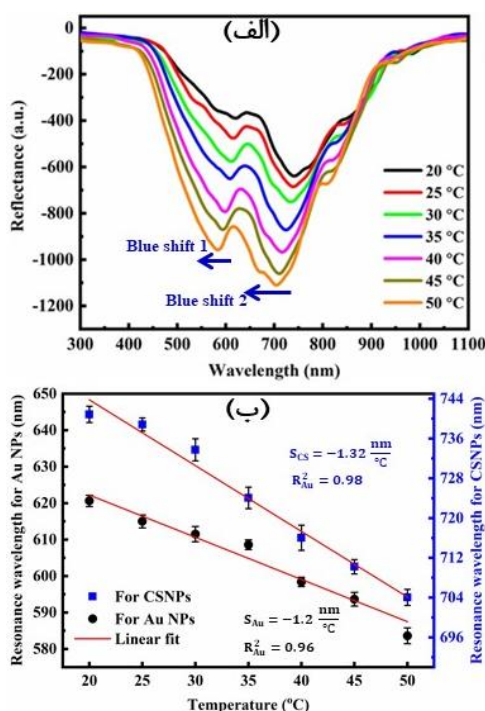
شکل ۹: (الف) طیف های بازتابی و (ب) \lambda_{res} حسگرعامل دار به نانوذرات ترکیبی CSNPs و NPs Au در بازه ۲۰-۵۰ °C.
