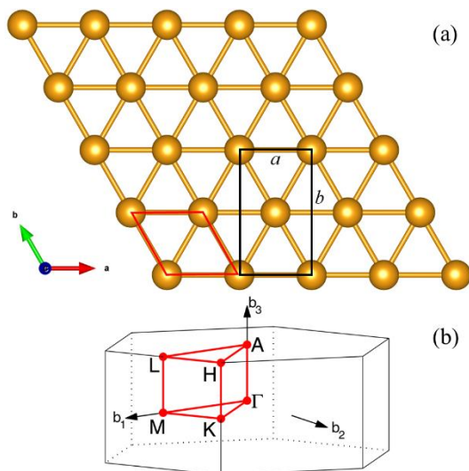
شکل ۱: (a) ساختار بلوری تک لایه Cu, Ag و Au. لوزی قرمز رنگ سلول واحد پیشنهادی در این پژوهش. مستطیل مشکی، سلول واحد در نظر گرفته شده در مطالعات پیشین. (b) منطقه اول بریلوئن برای ساختار شش گوشه و مسیر پر تقارن \Gamma - M - K - \Gamma .
