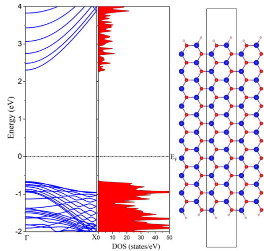
شکل ۱: ساختار کریستالی، ساختار نواری انرژی و چگالی حالات کل ترکیب خالص نانونوار AlN مورد بررسی.
