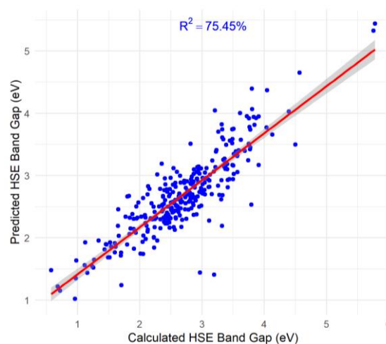
شکل ۲: نتایج حاصل برای یادگیری ماشین با در نظر گرفتن تمامی پارامترهای اتمی
