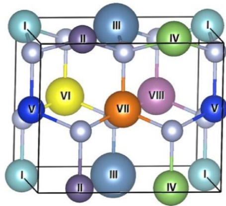
شکل ۱: ساختار کریستالی ترکیب در نظر گرفته شده و جایگاه های تفاوت اتمی برای آلاییدن یون های مورد نظر.
