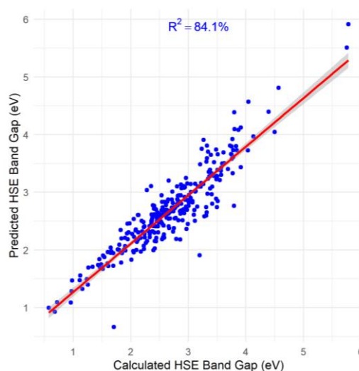
شکل ۳: نتایج حاصل برای یادگیری ماشین با در نظر گرفتن تمامی پارامترهای اتمی به علاوه انرژی نواری
