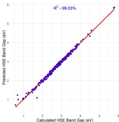
شکل ۹: نتایج حاصل برای یادگیری ماشین در نظر گرفتن تمامی پارامترهای اتمی و کریستالی
