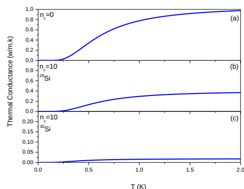
شکل (۵) - رسانندگی گرمایی نانو سیم سیلیکون (a) بدون ناخالصی ( n_c = 0 ) در حضور ناخالصی ^{29}\text{Si} ( n_c = 10 ) (b) در حضور ناخالصی ^{30}\text{Si} ( n_c = 10 ) (c)
