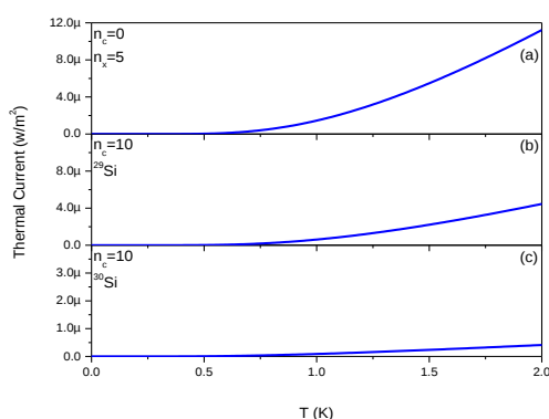
شکل (۶) جریان گرمایی نانو سیم سیلیکون - (a) بدون ناخالصی - (b) در حضور ناخالصی ^{29}\text{Si} ( n_c = 10 ) - (c) در حضور ناخالصی ^{30}\text{Si} ( n_c = 10 )
