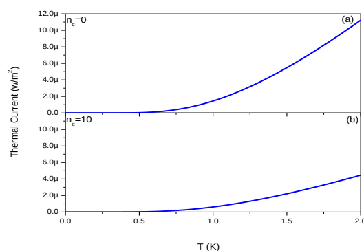
شکل (۴) - جریان گرمایی نانو سیم سیلیکون - (a) بدون ناخالصی - (b) در حضور ناخالصی ^{29}\text{Si} ( n_c = 10 )
