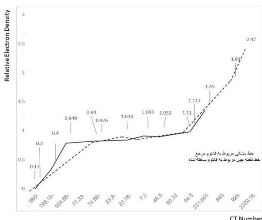
شکل ۵. منحنی های CT-ED فانتوم مرجع و فانتوم ساخته شده.
