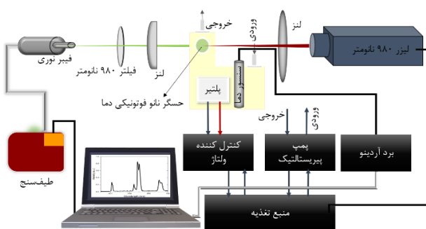
شکل ۱: چیدمان اپتیک، شدت تابش برای نظارت بر تغییرات دما
