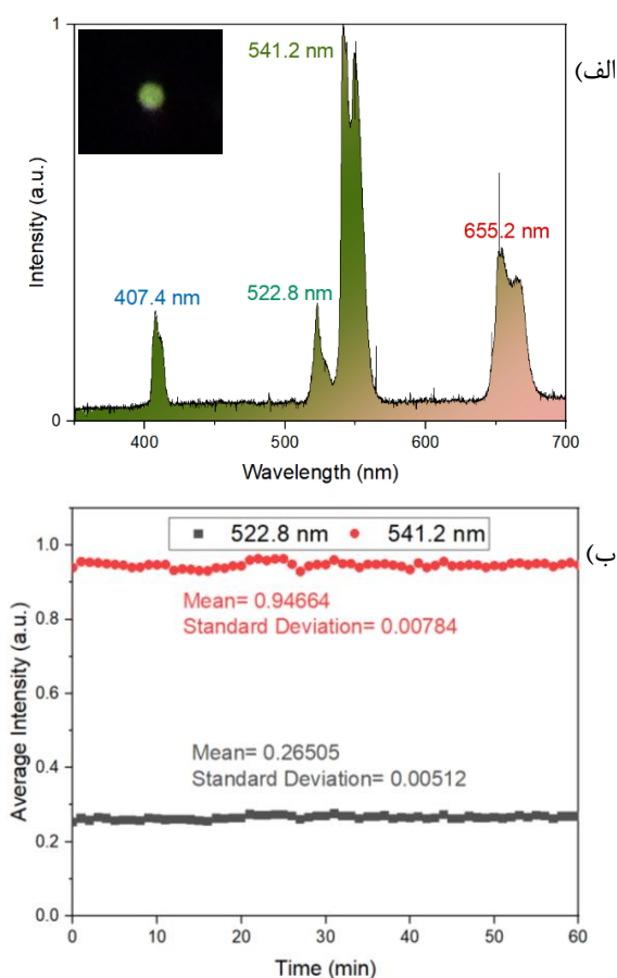
شکل ۳: (الف) نمودار PL نانوذرات (ب) نمودار پایداری تابشی طول موج ۵۲۲٫۸ و ۵۴۱٫۲ نانومتر
