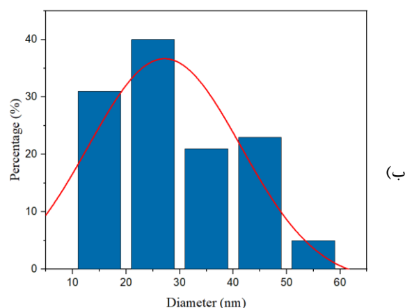
شکل ۲: (الف) تصویر TEM نانوذرات هسته-پوسته تبدیل‌افزایشی (ب) نمودار توزیع اندازه نانوذرات \text{Ba}_2\text{LuF}_7:\text{Yb}^{3+}, \text{Nd}^{3+}, \text{Er}^{3+}@\text{Ba}_2\text{LaF}_7
