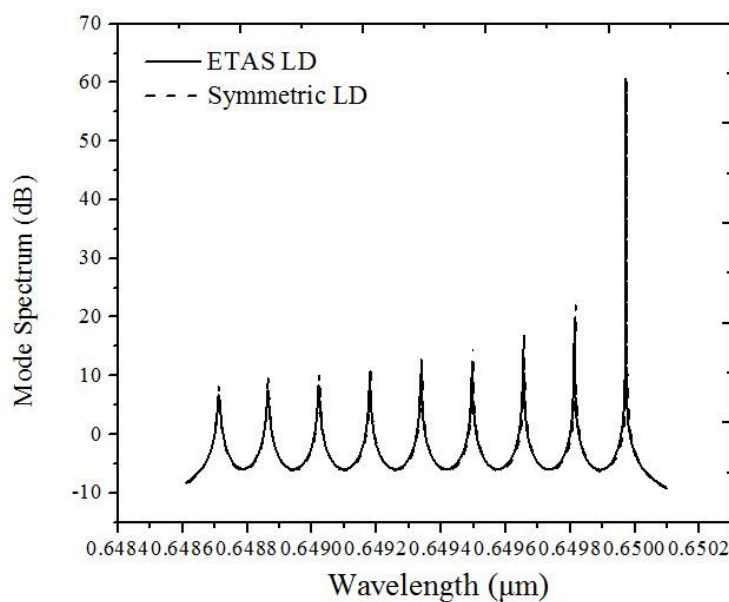
شکل ۳. طیف های مد لیزر متقارن و لیزر ETAS در ۲۰۰ mA و دمای زمینه ۲۰°C
