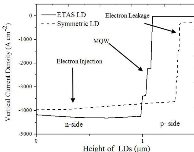
شکل ۸. چگالی جریان الکترون شبیه سازی شده بر حسب ارتفاع برای ساختارهای متقارن و ETAS در جریان تزریقی ۲۰۰mA و دمای زمینه ۲۰°C
