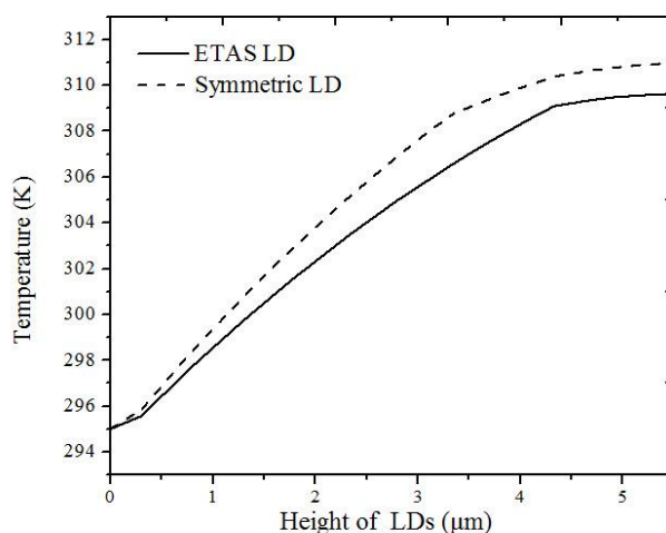
شکل ۹. نمودارهای دمایی محاسبه شده بر حسب ارتفاع برای ساختارهای متقارن و ETAS در جریان تزریقی ۲۰۰ mA و دمای زمینه ۲۰°C
