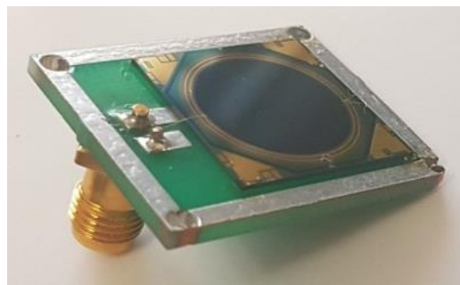
شکل ۳. آشکارساز تابش سیلیکونی PIN ساخته شده با سطح ناحیه‌ی حساس 163 \text{ mm}^2 بعد از نصب بر روی سازه‌ی مناسب برای انجام تست‌ها الکترونیکی و طیف سنجی تابش آلفا.
