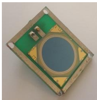
شکل ۳. آشکارساز تابش سیلیکونی PIN ساخته شده با سطح ناحیه‌ی حساس 163 \text{ mm}^2 بعد از نصب بر روی سازه‌ی مناسب برای انجام تست‌ها الکترونیکی و طیف سنجی تابش آلفا.
