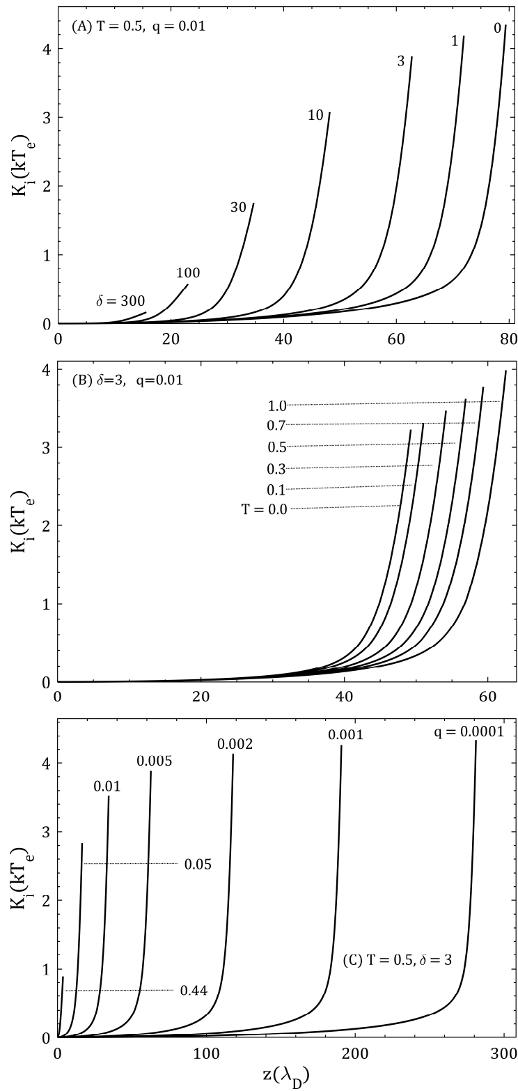
شکل ۳ توزیع انرژی جنبشی نرمالیزه شده یون K_i (با پارامتر نرمالیزاسیون kT_e = 1 eV بر حسب ضخامت لایه مرزی نرمالیزه شده Z (با پارامتر نرمالیزاسیون \lambda_D = 5/259 \times 10^{-7} m). تمام دیگر پارامترها با پارامترهای موجود در شکل ۲ یکسان است.
