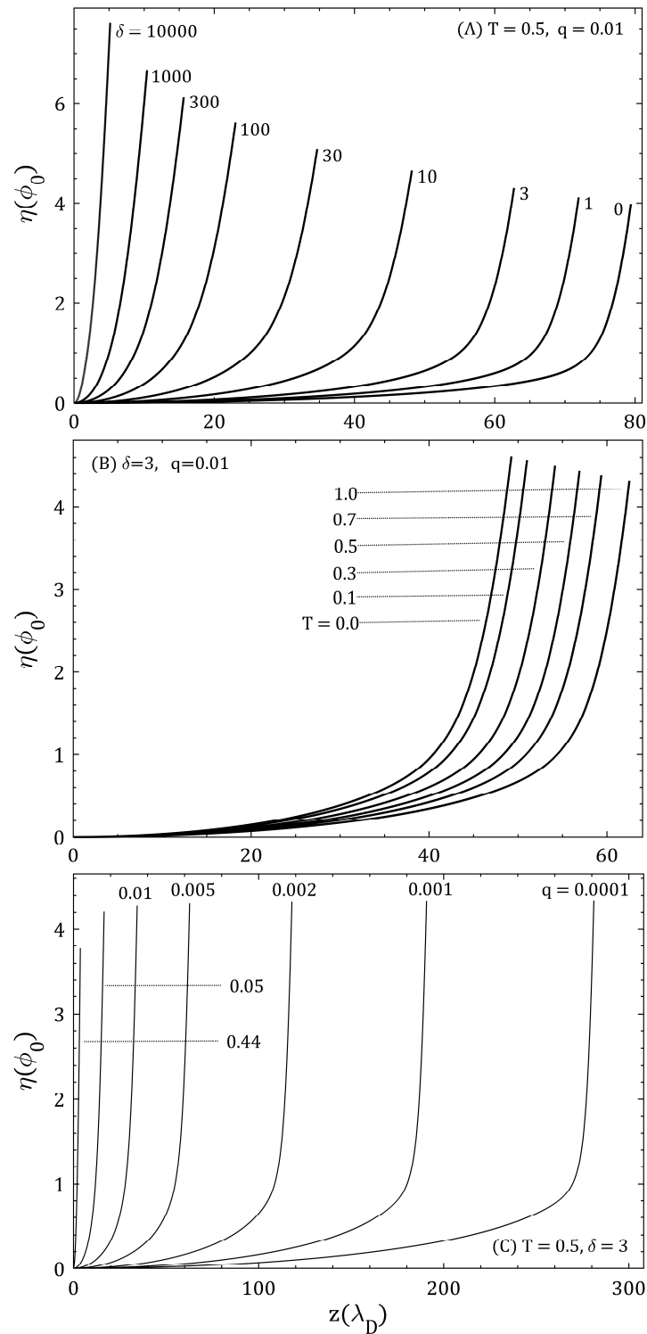
شکل ۲. توزیع پتانسیل الکتریکی نرمالیزه شده \eta (با پارامتر نرمالیزاسیون \phi_0 = kT_e/e = 1 V بر حسب ضخامت لایه مرزی نرمالیزه شده Z (با پارامتر نرمالیزاسیون \lambda_D = 5.259 \times 10^{-7} m به ازای، T = 0.5, q = 0.01 (A) و برخوردهای کشسان متفاوت \delta ، \delta = 3 (B) و دماهای متفاوت یون T و q = 0.01 (C) و T = 0.5, \delta = 3 و آهنگهای یونیواسیون متفاوت q .
