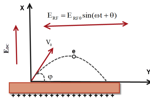
شکل ۱: مدل مالتی پکتینگ تک سطحی در دی الکتریک ها.
