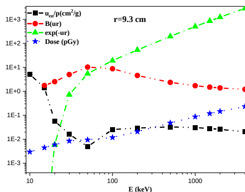
شکل (۶): نمودار تغییرات دز و عوامل موثر بر آن بر حسب انرژی فوتون در r=9.3 \text{ cm}
