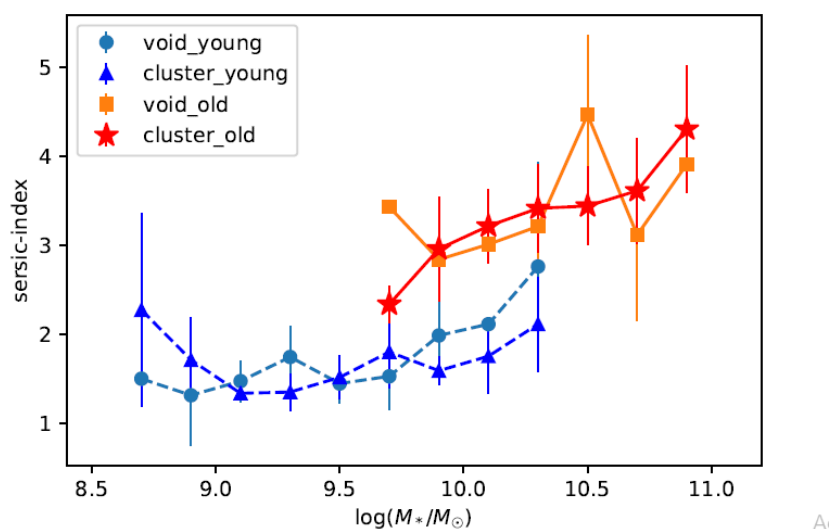
شکل ۵. نمودار تغییرات شاخص سرسیک برحسب جرم ستاره‌ای کهکشان‌های پیر و جوان در دو محیط مختلف
