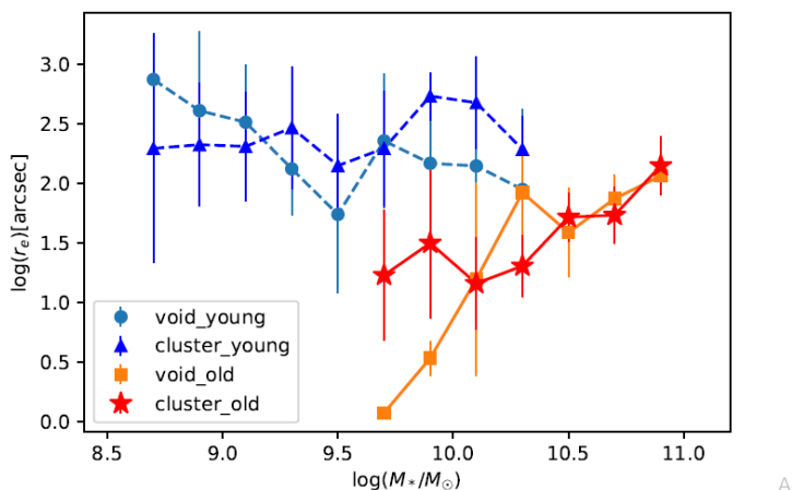
شکل ۳. نمودار تغییرات اندازه کهکشان (شعاع مؤثر) برحسب جرم ستاره‌ای کهکشان‌های پیر و جوان در دو محیط مختلف
