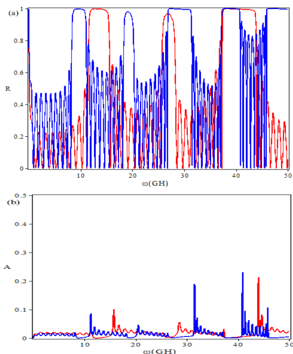
شکل ۶. اثر گذردهی نسبی لایه‌های دی‌الکتریک بر (a) انعکاس و (b) جذب برای \epsilon_{d1} = 2.1 (قرمز)، \epsilon_{d1} = 4.2 (آبی) و \epsilon_{d2} = 8
