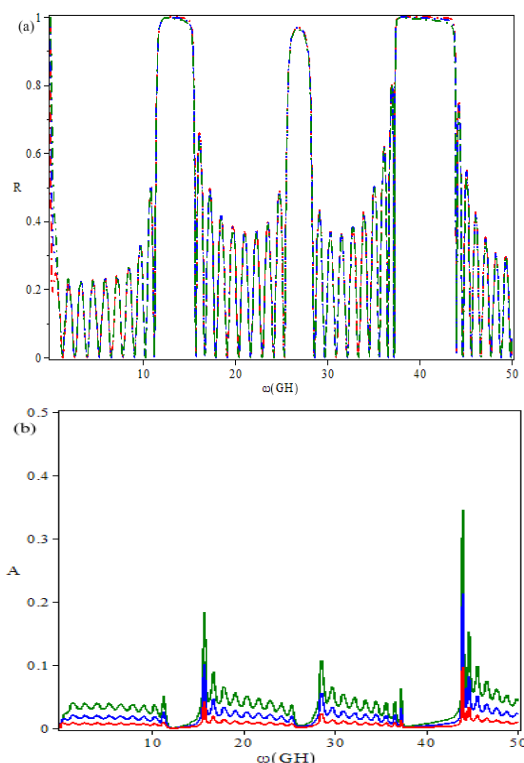
شکل ۲. اثر دماهای متفاوت الکترونی لایه‌های پلاسما بر (a) انعکاس و (b) جذب در \tau = 0.002 (قرمز)، 0.005 (آبی)، 0.01 (سبز)
