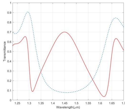
شکل ۲. قرمز رنگ (پیوسته): طیف عبور ساختار با بازتاب دهنده براگ و بدون تشدیدگر مستطیلی، آبی رنگ (خط چین): طیف عبور بازتاب دهنده براگ تعبیه شده در موجبر اصلی. پارامترهای مورد استفاده: w=50nm ، g_1=80nm ، g_2=100nm و d_1=d_2=285nm
