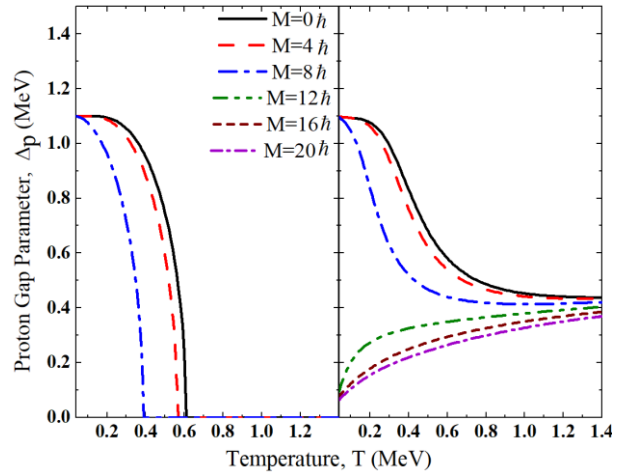
شکل ۵: پارامتر گاف پروتونی بر حسب دما در تکانه‌های زاویه‌ای مختلف برای هسته ^{147}\text{Nd} . سمت چپ: مدل BCS؛ سمت راست: مدل MEGBCS.
