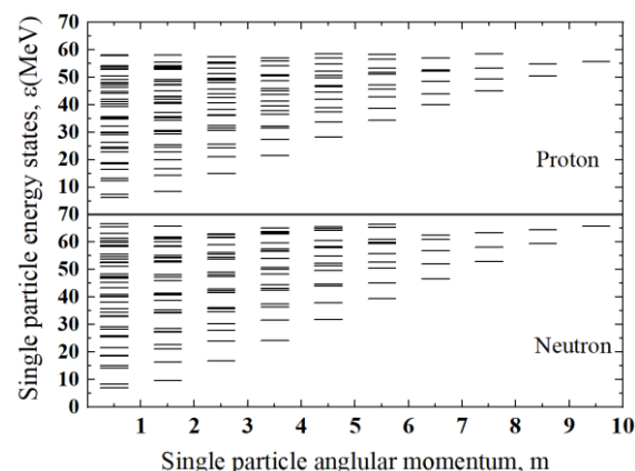
شکل ۲: ترازهای انرژی تک‌ذره‌ای پروتونی و نوترونی بر حسب اسپین برای هسته ^{146}\text{Nd} .
