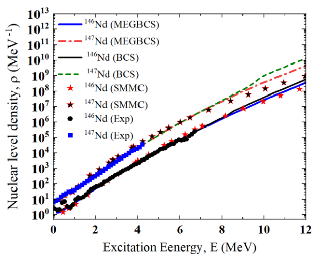
شکل ۱۵: چگالی تراز هسته‌ای بر حسب انرژی برانگیختگی در تکانه زاویه‌ای J = 0 \hbar در دو مدل BCS و MEGBCS برای هسته‌های ^{146}\text{Nd} و ^{147}\text{Nd} . داده‌های تجربی و نتایج مدل SMMC از مرجع [۲۵] اخذ شده‌اند.
