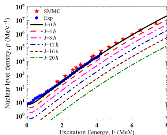
شکل ۱۴: چگالی تراز هسته‌ای بر حسب انرژی برانگیختگی در تکانه‌های زاویه‌ای مختلف برای هسته ^{147}\text{Nd} . داده‌های تجربی و نتایج مدل SMMC از مرجع [۲۵] اخذ شده‌اند.
