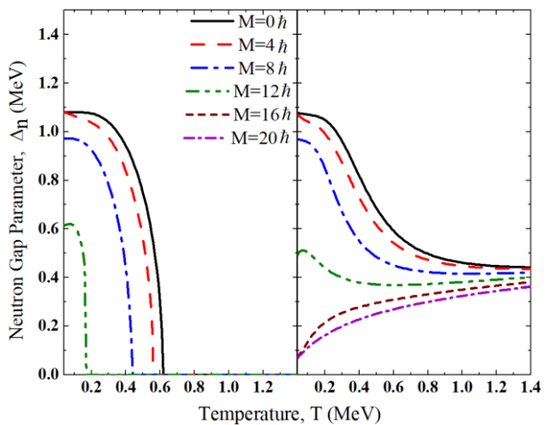
شکل ۶: پارامتر گاف نوترونی بر حسب دما در تکانه‌های زاویه‌ای مختلف برای هسته ^{147}\text{Nd} . سمت چپ: مدل BCS؛ سمت راست: مدل MEGBCS.
