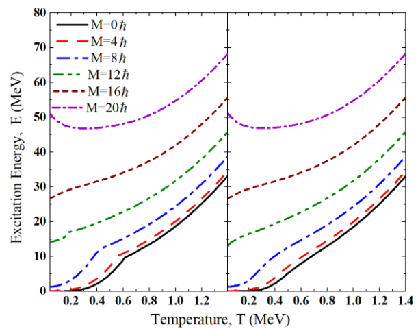
شکل ۹: انرژی برانگیختگی بر حسب دما در تکانه‌های زاویه‌ای مختلف برای هسته ^{147}\text{Nd} . سمت چپ: مدل BCS؛ سمت راست: مدل MEGBCS.
