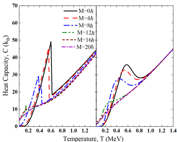
شکل ۱۲: ظرفیت گرمایی بر حسب دما در تکانه‌های زاویه‌ای مختلف برای هسته ^{147}\text{Nd} . سمت چپ: مدل BCS؛ سمت راست: مدل MEGBCS. ثابت بولتزمن می‌باشد.
