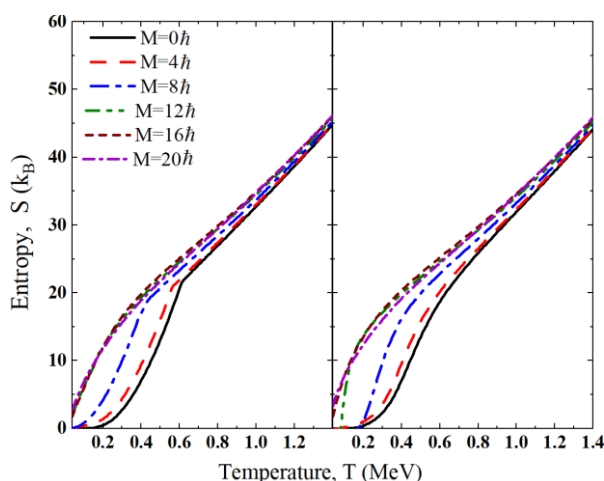
شکل ۸: آنتروپی بر حسب دما در تکانه‌های زاویه‌ای مختلف برای هسته ^{147}\text{Nd} . سمت چپ: مدل BCS؛ سمت راست: مدل MEGBCS. k_B ثابت بولتزمن می‌باشد.
