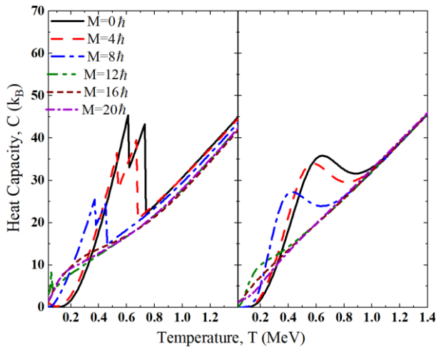
شکل ۱۱: ظرفیت گرمایی بر حسب دما در تکانه‌های زاویه‌ای مختلف برای هسته ^{147}\text{Nd} . سمت چپ: مدل BCS؛ سمت راست: مدل MEGBCS. ثابت بولتزمن می‌باشد.
