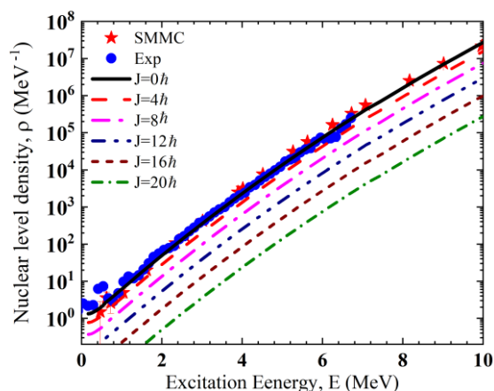
شکل ۱۳: چگالی تراز هسته‌ای بر حسب انرژی برانگیختگی در تکانه‌های زاویه‌ای مختلف برای هسته ^{146}\text{Nd} . داده‌های تجربی و نتایج مدل SMMC از مرجع [۲۵] اخذ شده‌اند.
