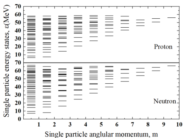
شکل ۱: ترازهای انرژی تک‌ذره‌ای پروتونی و نوترونی بر حسب اسپین برای هسته ^{146}\text{Nd} .
