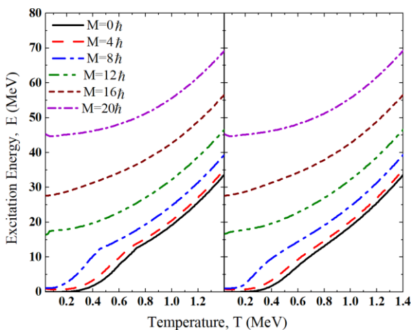
شکل ۷: انرژی برانگیختگی بر حسب دما در تکانه‌های زاویه‌ای مختلف برای هسته ^{146}\text{Nd} . سمت چپ: مدل BCS؛ سمت راست: مدل MEGBCS.
