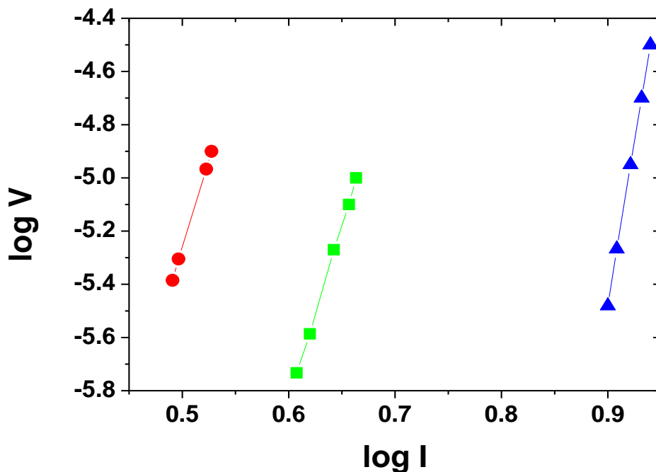
شکل ۷. نمودار \log V - \log I برای نمونه آلیش داده شده با مقدار Pb و Sb به مقدار y = 0.05 و x = 0.25 با زمان های پخت ۱۵۰، (۰٫۲۷) و ۲۷۰ (۰٫۲۷) ساعت
