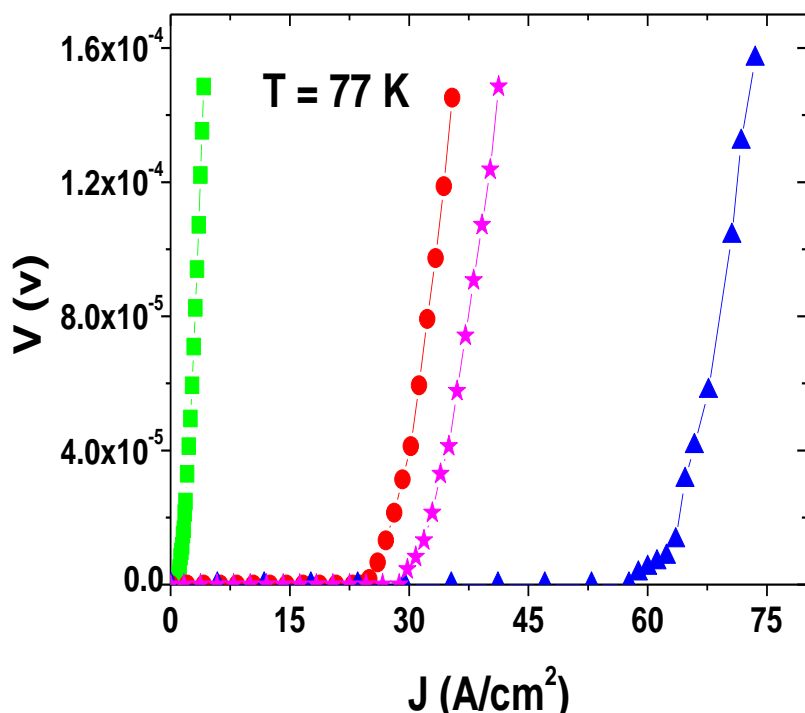
شکل ۳. نمودارهای V - J برای مقادیر متفاوت Pb و Sb : (\blacktriangle) 0.35 ، (\bullet) 0.36 ، (\blacksquare) 0.4 ، (\star) 0.32 با زمان پخت ۲۷۰ ساعت و 0.08 و 0.35 ، 0.05 ، 0.36 ، 0.04 ، 0.0 .
