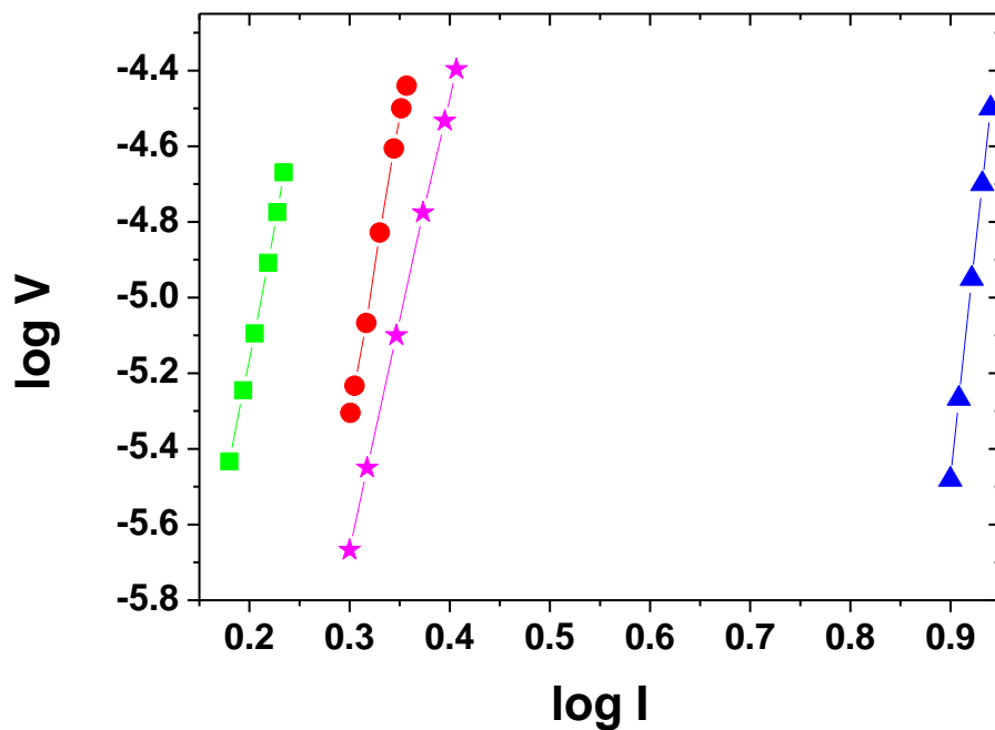
شکل ۶. نمودار \log V - \log I برای نمونه‌های آلیش داده شده با مقادیر مختلف Pb و Sb: \square (۰٫۰۲)، \bullet (۰٫۲۸)، \blacktriangle (۰٫۰۵)، \circ (۰٫۳۵)، \star (۰٫۲۰، ۰٫۳۰) و \star (۰٫۲۰، ۰٫۳۰) با زمان پخت ۲۷۰ ساعت.
