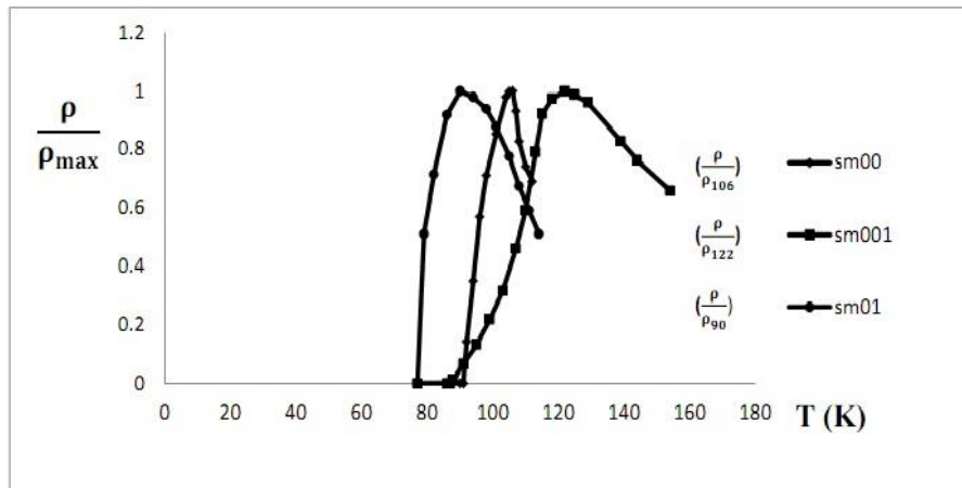
شکل ۱۱. نمودار مقایسه‌ای مقاومت ویژه بر حسب دمای نمونه‌های خالص و آلییده SBCO.
