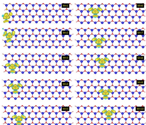
شکل ۵: چگالی الکترونی اسپین قطبیده سه بعدی برای تمامی پیکربندی های آلاییده با اتم منگنز. مقدار واحد هم خط برای رسم چگالی برابر 10^{19} می باشد.
