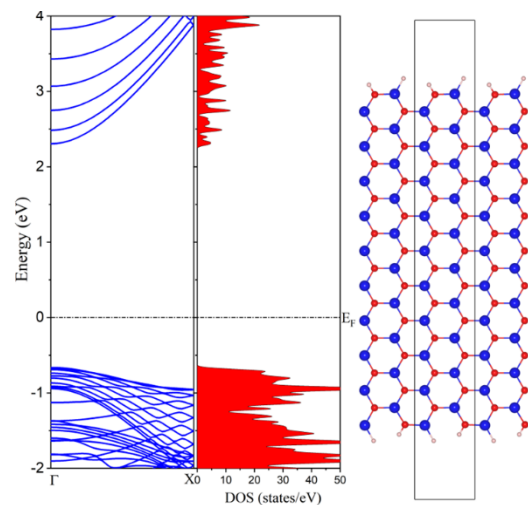
شکل ۱: ساختار کریستالی، ساختار نواری انرژی و چگالی حالت کل ترکیب خالص نانونوار AlN مورد بررسی.
