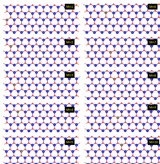
شکل ۶: ساختار کریستالی نانونوارهای آلاییده با اتم منگنز
