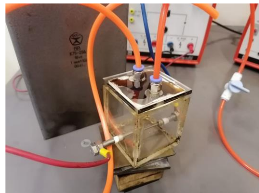
شکل ۱: نمای راکتور و الکتروودها
