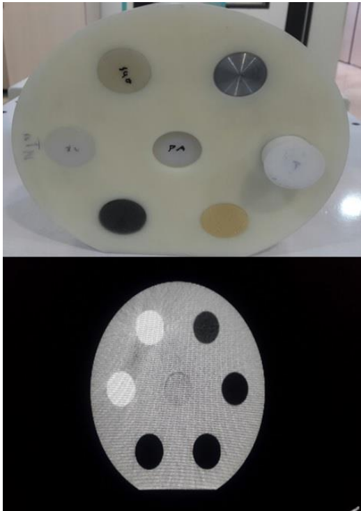
شکل ۳. تصویری از فانتوم ساخته شده. بالا: نمایی از فانتوم ساخته شده، پایین: تصویر سی تی فانتوم ساخته شده.
