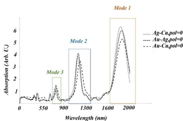
شکل ۲: مدهای مختلف سطح مقطع جذب نانوذرات دوتایی ناهمگن از جنس Au-Cu و Ag-Cu و Au-Ag.
