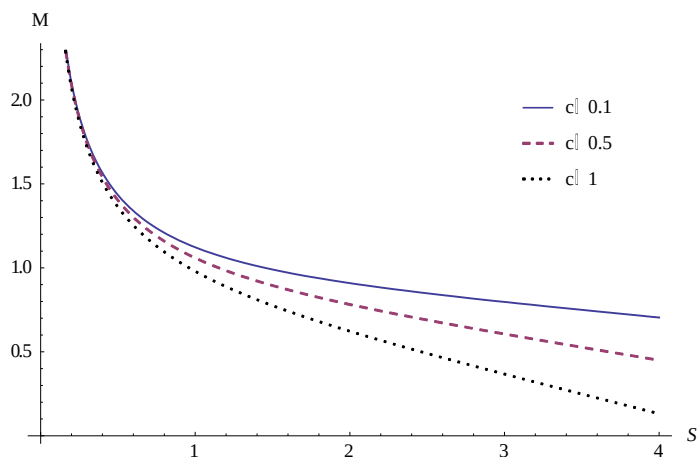
شکل ۵. نمودار تغییرات جرم بر حسب آنتروپی به ازای مقادیر مختلف c و Q = 1 ، \Lambda = 1
