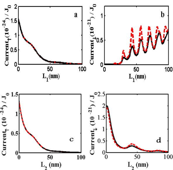
شکل ۲: چگالی جریان اسپینی در ساختار پنج لایه‌ای
