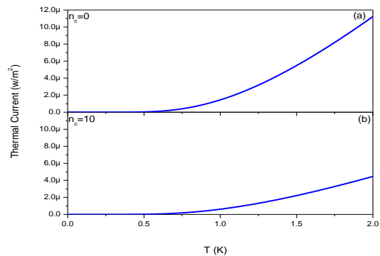
شکل (۴) - جریان گرمایی نانو سیم سیلیکون - (a) بدون ناخالصی - (b) در حضور ناخالصی ^{29}Si ( n_c = 10 )
