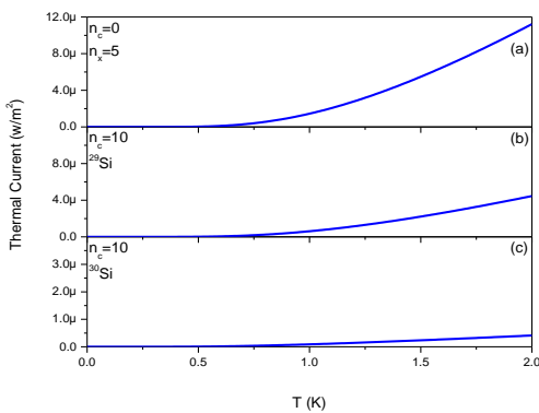
شکل (۷) - جریان گرمایی نانو سیم سیلیکون - (a) بدون ناخالصی - (b) در حضور ناخالصی ^{29}Si ( n_c = 10 ) - (c) در حضور ناخالصی ^{30}Si ( n_c = 10 )
