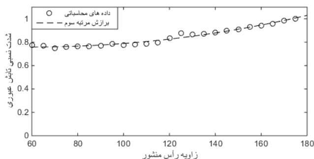
شکل ۹. نمودار رابطه شدت تابش نسبی عبوری (انتگرال ضریب عبور بر حسب زاویه تابش) با زاویه رأس
