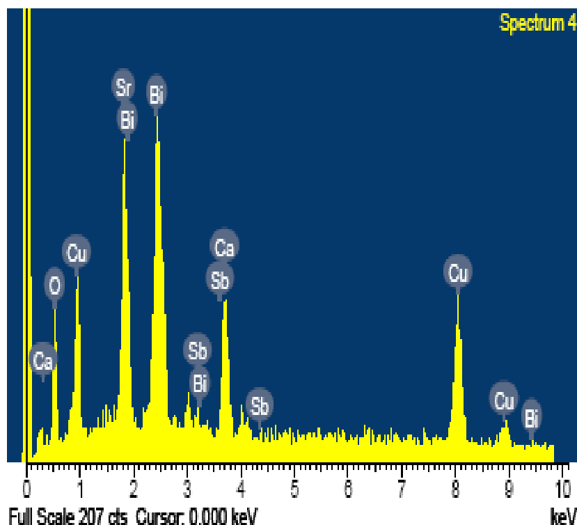
شکل ۹. تصویر EDX نمونه‌ای با Sb و Pb به مقدار y = 0.05 و x = 0.35 با زمان پخت ۲۷۰ ساعت.
