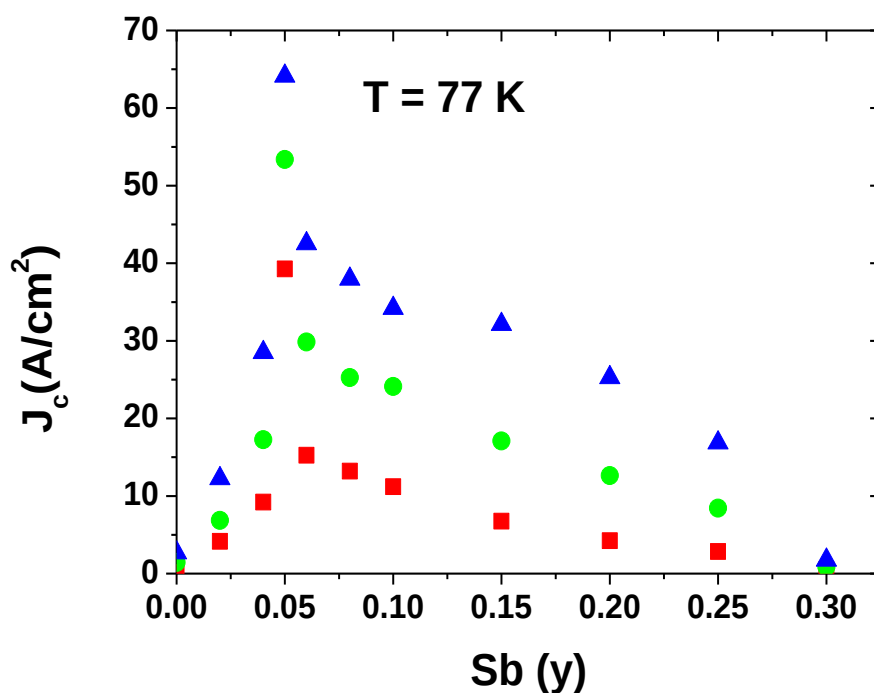
شکل ۴. چگالی جریان بحرانی نمونه‌های آلایش داده شده بر حسب مقادیر Sb و Pb با زمان‌های پخت ۱۵۰ ساعت (▲) ۲۷۰، (●) ۲۱۰، (■) ۹۰
