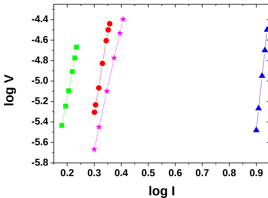
شکل ۶. نمودار \log V - \log I برای نمونه‌های آلیش داده شده با مقادیر مختلف Pb و Sb: \square (۰٫۰۲، ۰٫۳۸) \triangle (۰٫۰۵، ۰٫۳۵)، \bullet (۰٫۱۰، ۰٫۳۰) و \star (۰٫۲۰، ۰٫۲۰) با زمان پخت ۲۷۰ ساعت.
