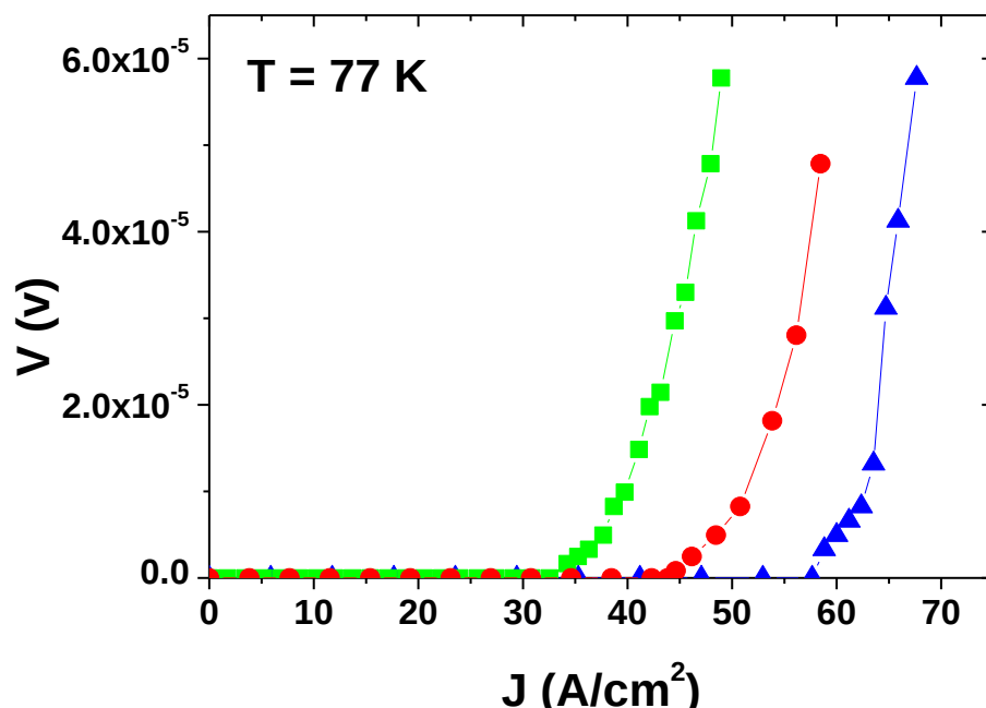
شکل ۲. نمودارهای V-J با زمان‌های پخت ۱۵۰، ۲۱۰ و ۲۷۰ ساعت برای نمونه‌ای با Sb و Pb به مقدار x = 0.35 و y = 0.5
