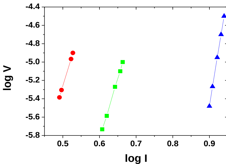
شکل ۷. نمودار \log V - \log I برای نمونه آلیش داده شده با Pb و Sb به مقدار y = ۰٫۰۵ و x = ۰٫۳۵ با زمان های پخت ۱۵۰، \square (۲۱۰)، \bullet (۲۷۰) و \triangle (۲۷۰) ساعت
