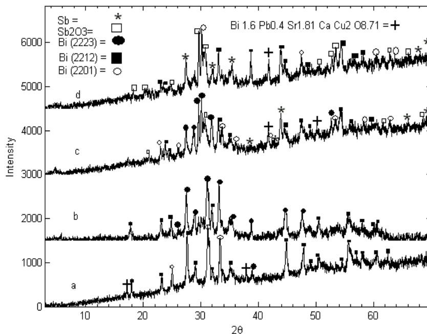
شکل ۱. الگوی پراش برای نمونه‌ها با مقدار Sb و Pb. a (۰٫۴، ۰٫۰)، b (۰٫۴۵، ۰٫۰۵)، c (۰٫۵، ۰٫۲۰)، d (۰٫۵، ۰٫۱۵) با زمان پخت ۲۷۰ ساعت
