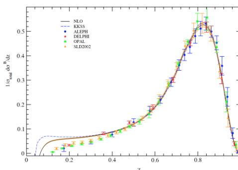
شکل ۳: مقایسه نتایج تئوری برای سطح مقطع دیفرانسیلی بهنجار شده (1/\sigma_{\text{tot}} \times d\sigma^B/dz) در مرتبه دوم اختلال با داده‌های آزمایشگاهی گزارش شده از گروه‌های ALEPH، DELPHI، OPAL و SLD. همچنین پیشگویی مدل‌مان (۸) در این مرتبه اختلال با پیشگویی مدل KKSS (نمودار خط-چین) [۶] در همین مرتبه مقایسه شده است.
