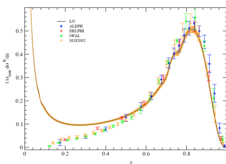
شکل ۲: مقایسه نتایج تئوری برای سطح مقطع دیفرانسیلی بهنجار شده (1/\sigma_{\text{tot}} \times d\sigma^B/dz) در مرتبه اول اختلال با داده‌های آزمایشگاهی گزارش شده از گروه‌های ALEPH، DELPHI، OPAL و SLD.
