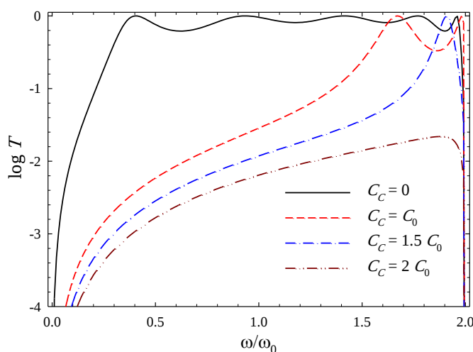
شکل ۴. ضریب عبور فونونی بر حسب بسامد فونون ورودی برای یک زنجیره‌ی جرم-فنر ساده شامل پنج یون متوالی مثبت و منفی که به دو هادی فونونی ساده متصل است، برای چند مقدار متفاوت C_C . در اینجا فرض شده است که جرم‌ها در کل سامانه با هم برابرند.
