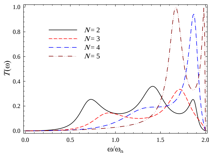
شکل ۵. ضریب عبور فونونی بر حسب بسامد فونون ورودی برای یک زنجیره‌ی جرم-فنر ساده پنج جرمی متصل به دو هادی فونونی ساده برای تعداد مختلف یون‌های مثبت و منفی متوالی در ابتدای سامانه‌ی مرکزی. در اینجا C_C = C_0 و جرم‌های سامانه یکسان فرض شده است.
